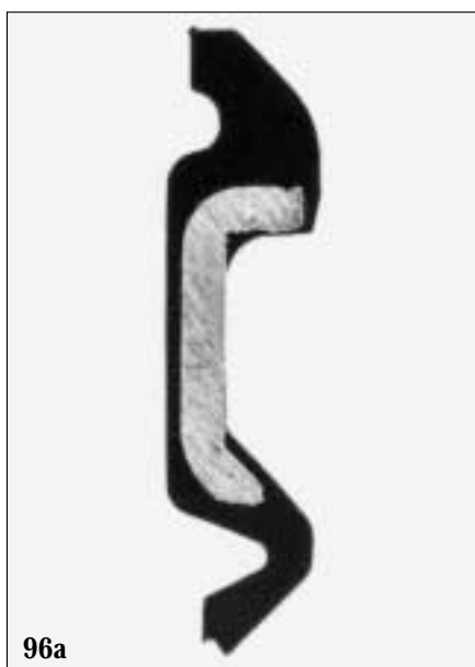
96: Sección transversal de una tapa de obturación a: labio de obturación nuevo; b: labio de obturación gastado
