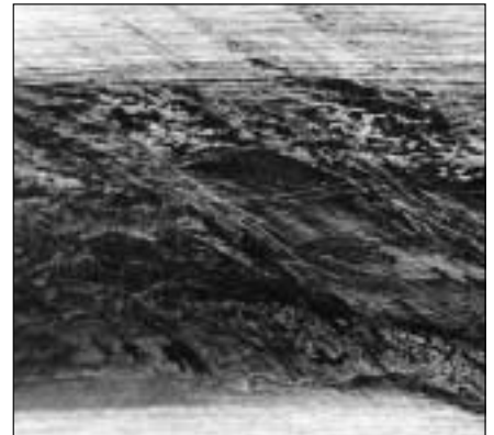
82: En la cara frontal de los rodillos y en el borde puede producirse desgaste por atascamiento en caso de suministro deficiente de lubricante y cargas elevadas.
